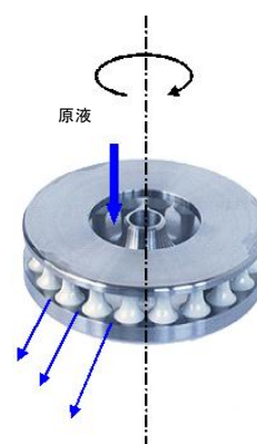
図 7 噴霧盤
